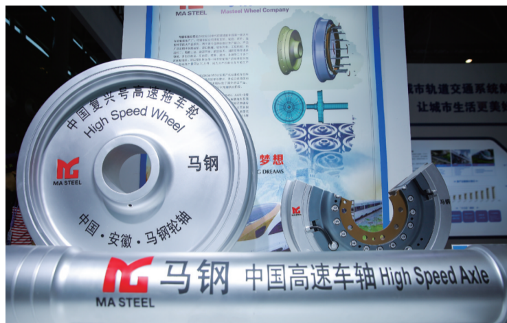
展馆内展示的复兴号高速拖车轮和车轴
