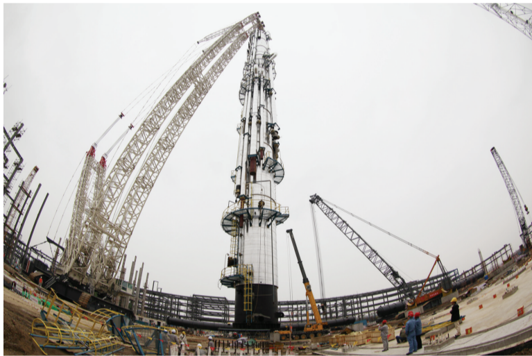
3月29日,中安联合煤化工项目再传模块化施工捷报,高度近百米的净化装置变换气吸收塔整体吊装一次成功。此次吊装的变换气吸收塔塔体长91.2米,直径达4米,是净化装置的关键设备,也是该装置实行模块化安装的首台大件设备。 ■ 陈海涛 记者 吴传贤 文/图
