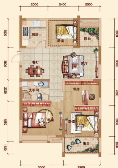
B 户型 2#楼 建筑面积约: 94.75平米 计一半建筑面积
