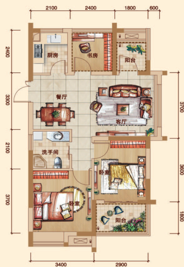
F 户型 6#楼 建筑面积约: 88.66平米 计一半建筑面积
